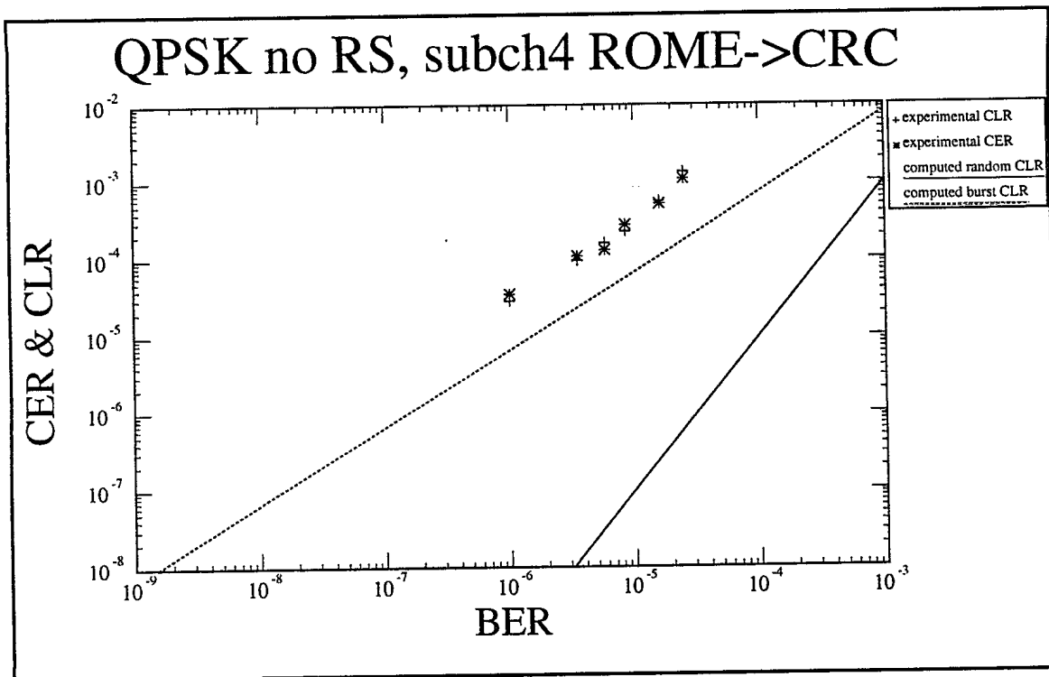
Figure8: QPSK subchannel 4DS0 Rome->CRC
